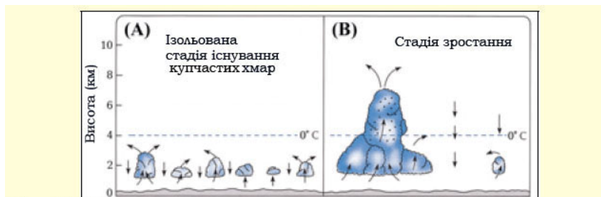
Мал. 19. (А) Ізольовані частинки купчастих хмар. (В) Коли маленькі хмари з'єднуються між собою, то починається формування великої хмари, яка зростає вертикально. Водяні краплі позначені крапками (The Atmosphere, Anthes and others, p. 269.). купчастих
