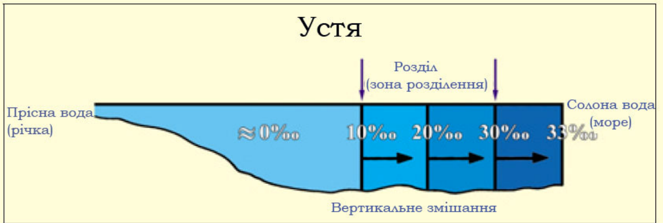
Мал. 14. Повздовжній розріз показує рівень солоності (тисячні ‰) в усті. Ми спостерігаємо розділ (зону розділення) між прісною і солоною водою. (Introductory Oceanography, Thurman, p. 301, з деякими доповненнями.)
