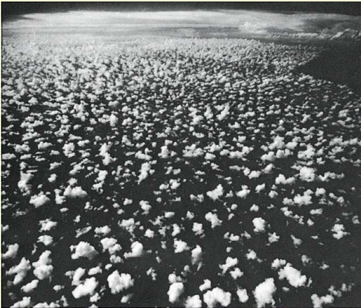
Мал. 18. Маленькі частинки хмар (купчасті хмари) рухаються в напрямі зони скупчення біля обрю, де ми можемо бачити велику дощову хмару. (Clouds and Storms, Ludlam, plate 7.4.)
